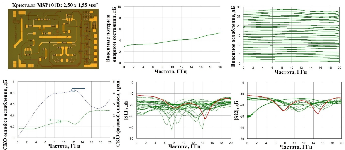
Рисунок 2. Топология кристалла и частотные характеристики MSP101D
