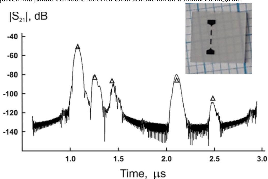
Рисунок1. Временной отклик трехдиапазонной РИМ.
