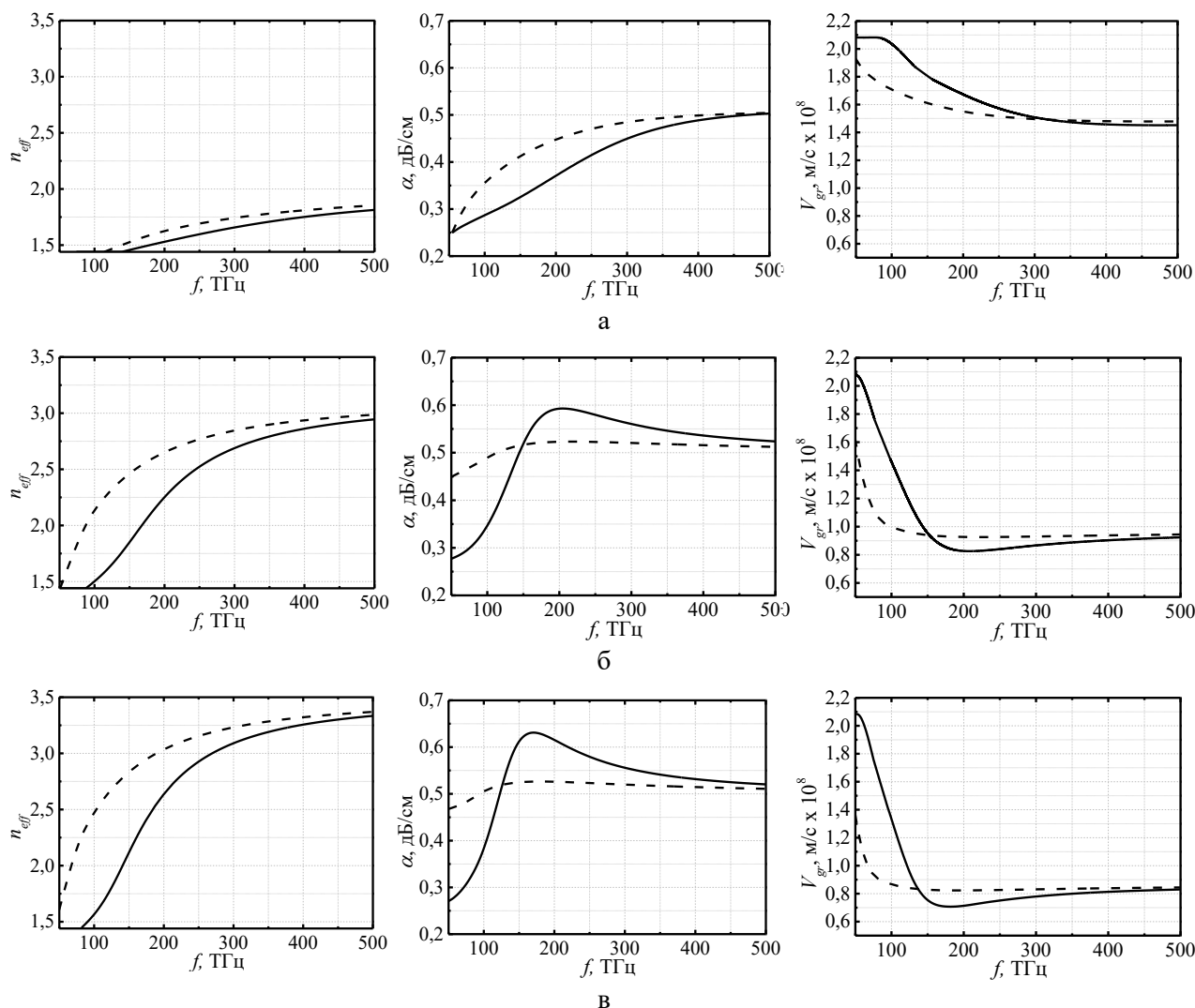
Рисунок 2. Частотные зависимости эффективного показателя преломления и значения собственных потерь в микроволноводе; сплошная линия соответствует E_y^{11} -моду, пунктирная – E_x^{11} .
