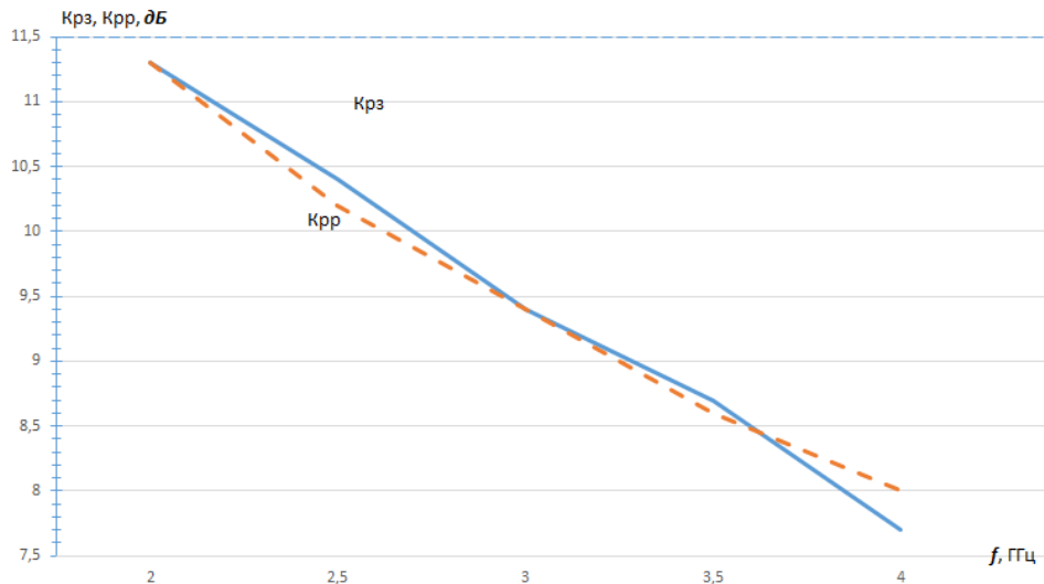
Рисунок 2. График зависимости K_{pz}(f) , K_{pp}(f)
