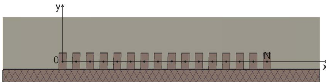
Рис. 1. Расположение нерезонансных щелей и эквивалентных точечных излучателей
