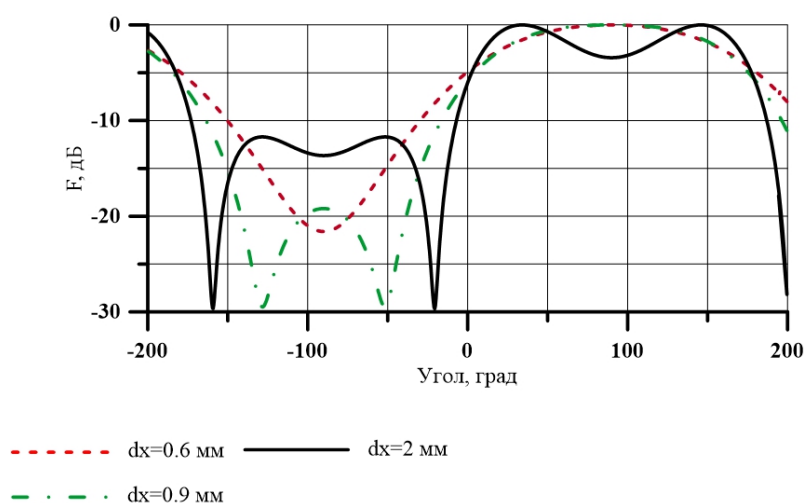
Рис.5. Результаты синтеза диаграммы направленности для антенны вытекающей волны
