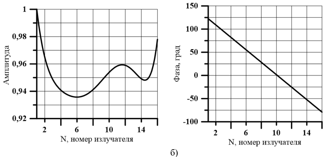
Рис. 2. Функции распределения амплитуды и фазы электромагнитного поля в антенне вытекающей волны
