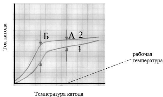
Рис. 5. Схема некокальных характеристик катодов в приборе: 1 – традиционные, 2 – плазменнонапыленные.
