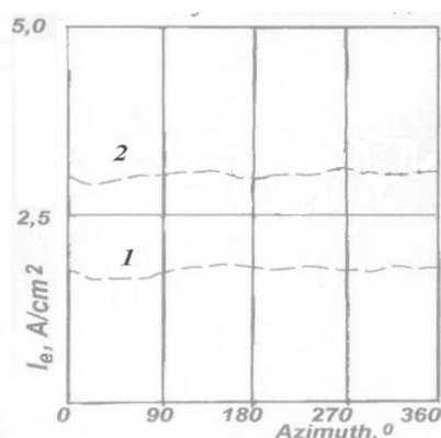
Рис. 4. Азимутальное распределение плотности тока для катода гиротрона
