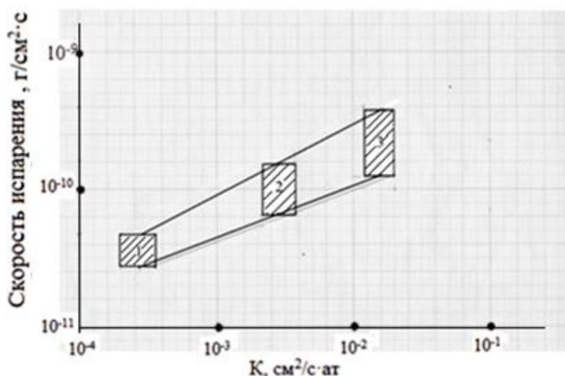
Рис. 3. Зависимость скорости испарения эмиссионного вещества
