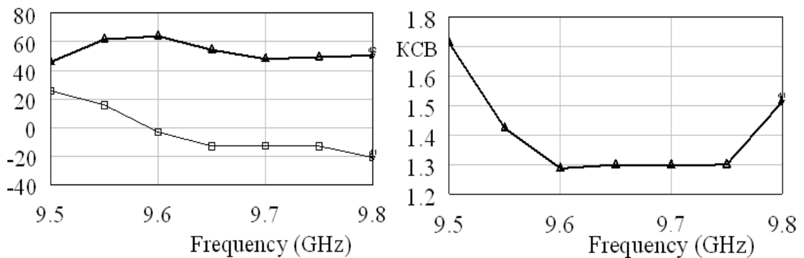
Рис.3. Активная ( R ) и реактивная ( X ) части входного сопротивления (а) и КСВ (б) по входу 2 с вертикальной поляризацией в диапазоне частот
