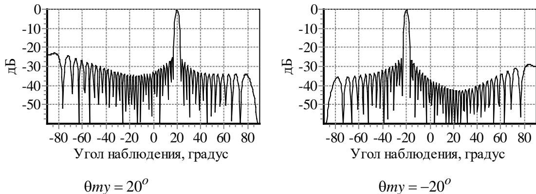
Рис.6. ДН в вертикальной плоскости для случая N_y=36 , шаг размещения излучателей D_y=21 мм, частота 9650 МГц
