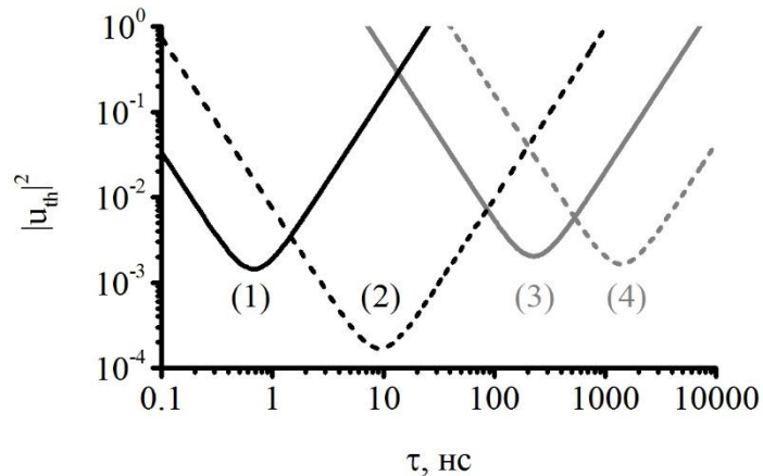
Рисунок 2. Пороги формирования солитонов СВ, распространяющихся в средах: (1) – пленке ВаМ, (2) – пленке ЖИГ, (3) – пленке ВаМ без учета обменного взаимодействия, (4) – пленке ЖИГ без учета обменного взаимодействия
