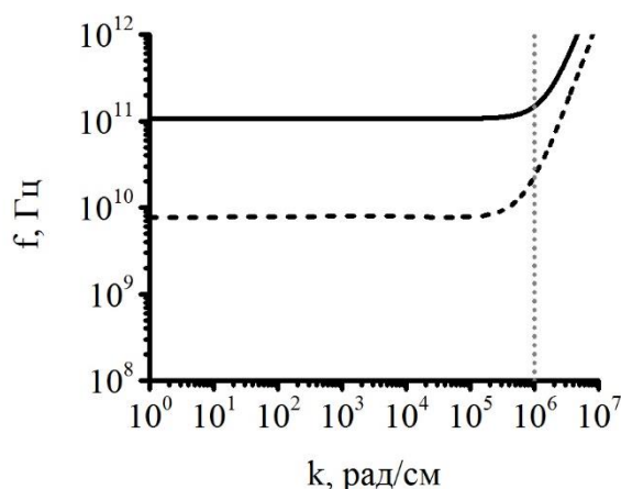
Рисунок 1. Дисперсионные характеристики СВ: в ВаМ – сплошная линия, в ЖИГ – штриховая линия (Значение волнового числа k = 10^6 рад/см – серая пунктирная линия.)
