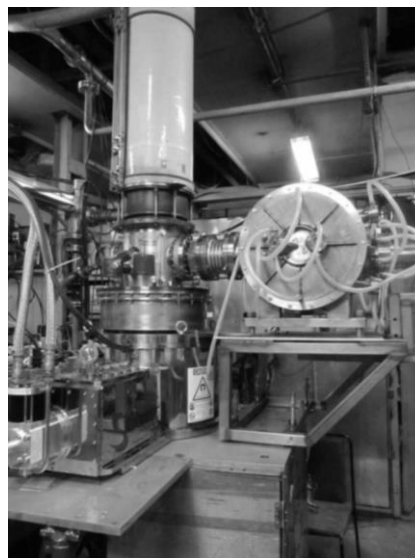
Рисунок 1. Гиротроны для ИТЭР в испытательных стендах со сверхпроводящими магнитами фирм CRYOMAGNETICS (USA) и JASTEC (Japan)
